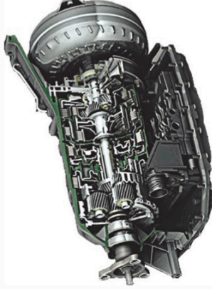
双离合变速器-DCT
