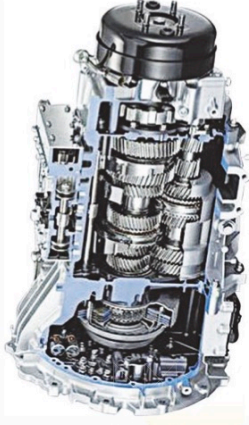
液力自动变速器-AT
